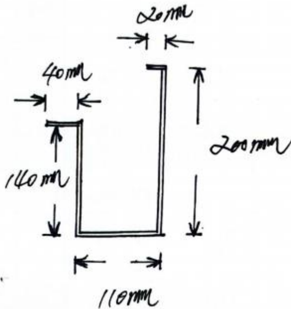
水沟槽制作尺寸 (附图)
